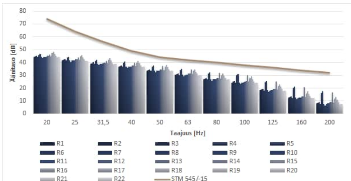
Kuva 3-2. Osayleiskaavasunnitelman mukaisen pientaajuisen melulaskennan tuloskuvaaja
