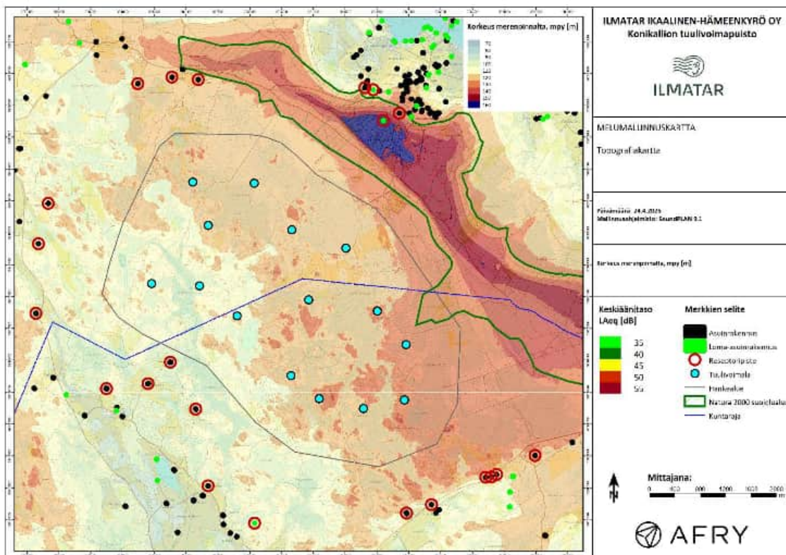
Kuva 2-1. Melumallinnuksen digitaalikarttan topografiamalli, mpy [m]
